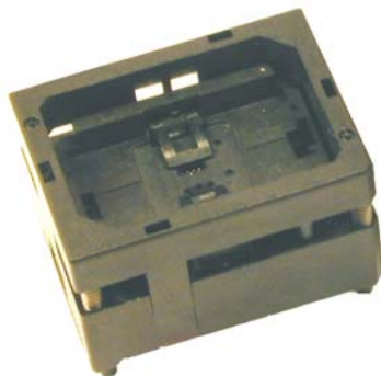
S-MBG-2X4-008-A Socket
